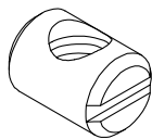
F (x2) Nut/Ecrou/Tuerca 3/8 x 1/4 x 4 1/2 in 9.5 x 6.35 x 13 mm
